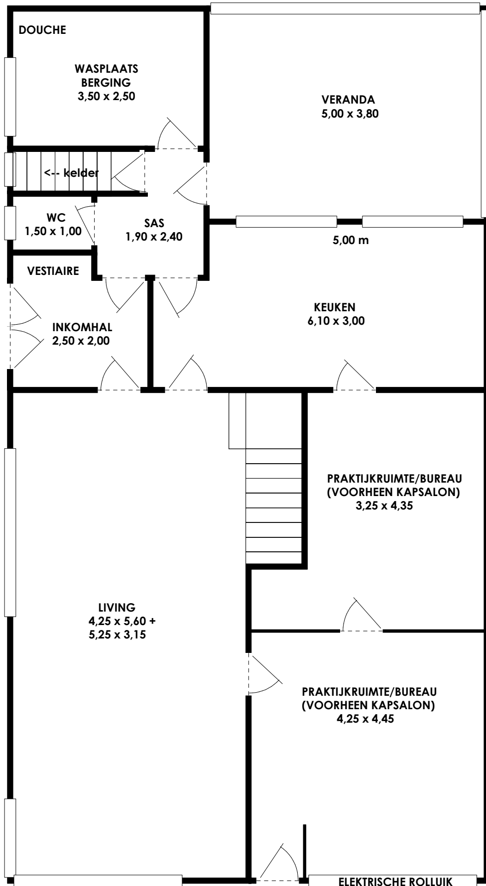
INDELINGSPLAN GELIJKVLOERS NOORD-ZUIDSTRAAT 3 KOERSEL
